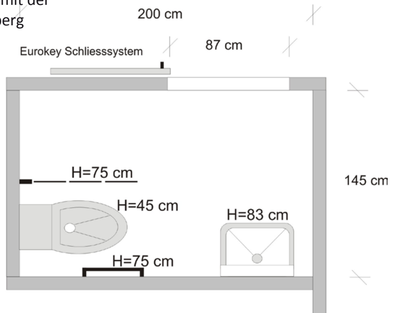
WC und Plan WC
